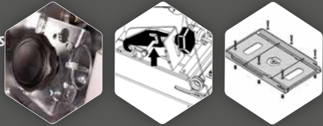
Snelwisselvoet voor snel uitwisselen tussen machines Plate for quick-change seeder between different implements Schnellwechselplatte für Wechsel mehreren Maschinen Plaque de changement pour monter sur une autre machine Sistema cambio rápido de Sembradora entre múltiples máq.
