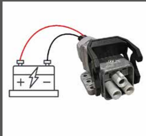
Kabel 5m voor stroomvoorziening direct vanaf accu tractor Cable for power supply directly from tractor battery Kabel für Stromversorgung direkt von der Traktorbatterie Câble d'électricité directement sur l'accu du tracteur Cable para alimentación directamente desde la tractorbatería
