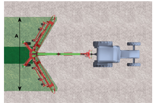
A = working width from 450 to 875 cm. A = largeur de travail de 450 à 875 cm.
